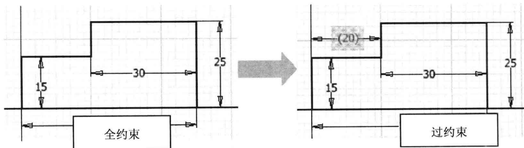
图 1-13 应用联动尺寸实例
