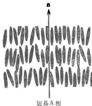
图 1.6 近晶 A 相和近晶 C 相的示意图
