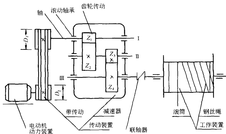
图 1-1 卷扬机传动示意图
