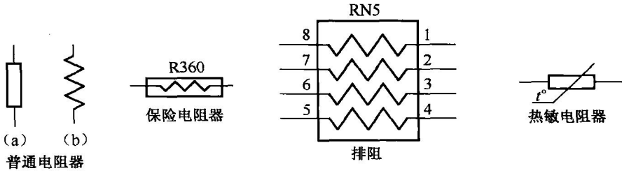
图 1-12 电路原理图中电阻器的符号
