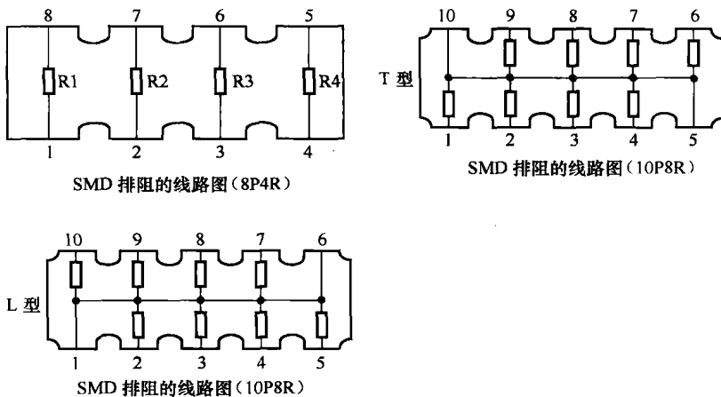
图 1-7 8P4R 和 10P8R 排阻的内部电路
