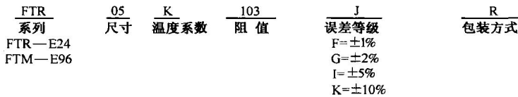
图 1-11 贴片电阻器的型号示意图
