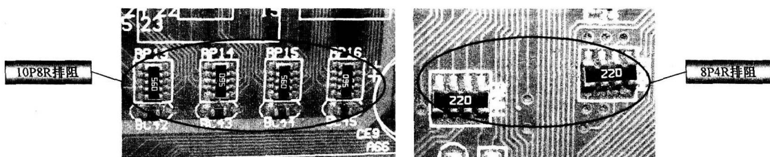
图 1-6 常见的贴片排阻
