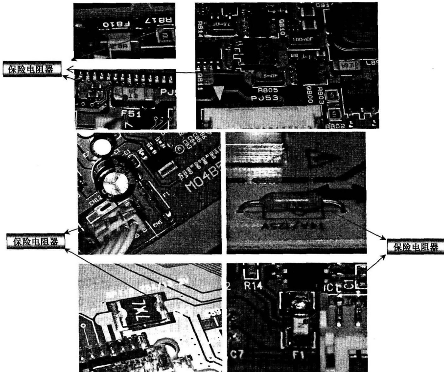
图 1-8 常用的贴片保险电阻器
