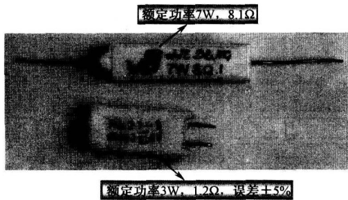
图 1-13 采用直标法标注的水泥电阻器示意图
