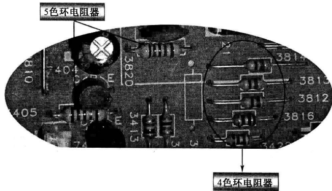
图 1-1 常用的色环电阻器
