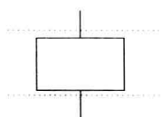
小阳线
