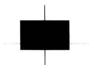
小阴线
