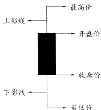
图1-2 阴线
