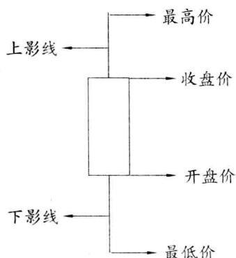
图1-1 阳线
