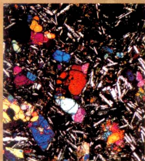
粗玄武岩 (在显微镜中利用偏光滤镜拍摄)
