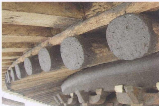
彩图3-7-3 老檐椽头、檐檩、压斗枋通灰
