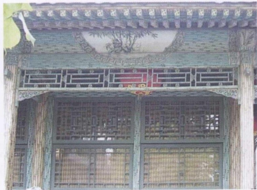
彩图4-1-3 斑竹座彩画
