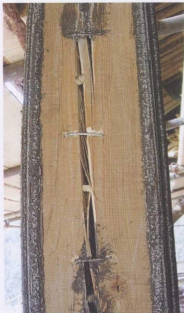
彩图3-4-1 下竹钉与扒锅子
