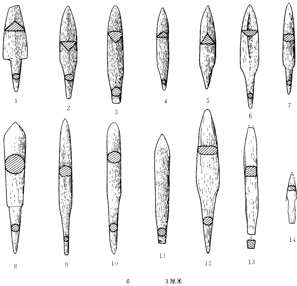
图四二一 商代二里岗下层二期骨镞
