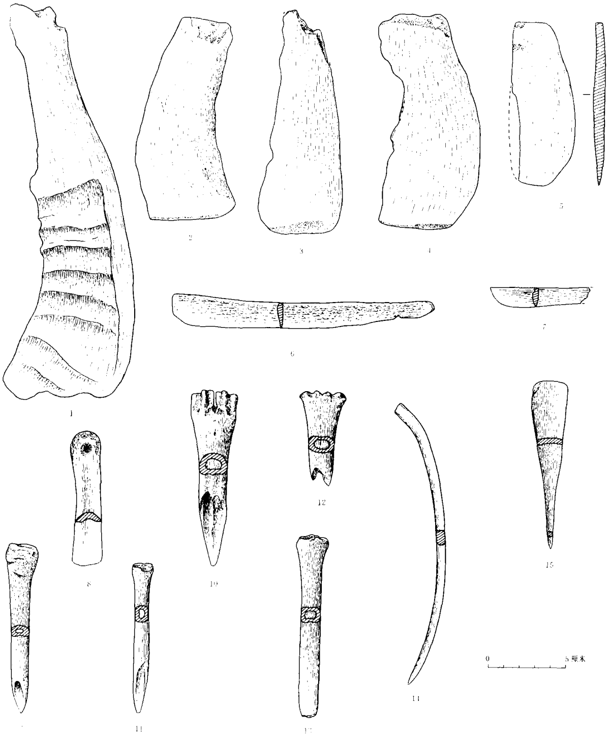
图四一九 南关外商代二里岗下层二期骨铲、刀、凿和锥
