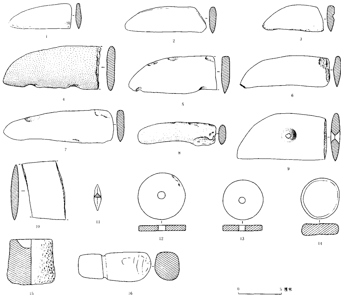
图四一七 商代二里岗下层二期石镰、戈、镞、纺轮、白和网坠
