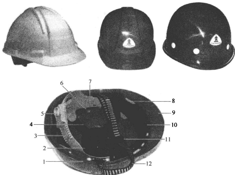
图 1-1 安全帽及其结构
