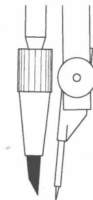
铅芯应磨成斜形， 针尖应稍长于笔尖
