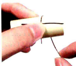
(2) 将铁丝竖放在套筒上，另取一根长短适中的铁丝与竖放的铁丝成十字形摆好。
