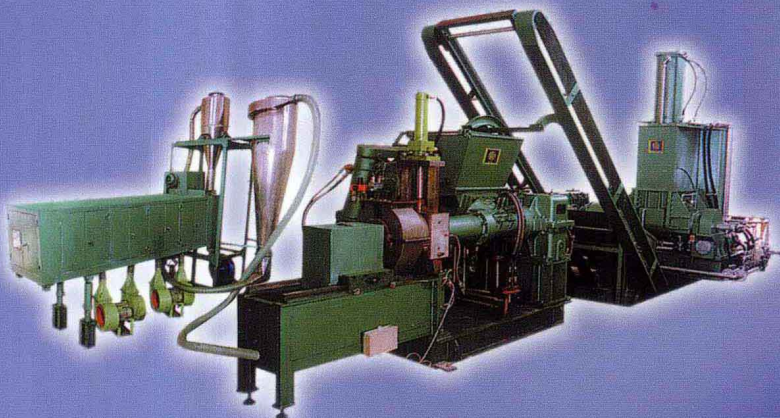
▲ 风冷式塑料造粒生产机组
