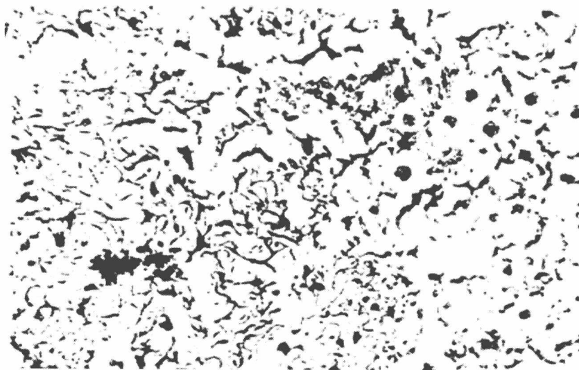
图 1-1 片状、蠕虫状、团状、球状石墨共存 [1]
