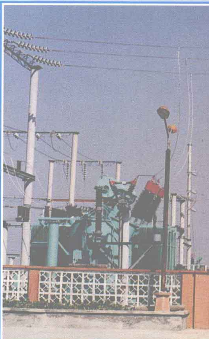
▼县城11万千伏变电站
