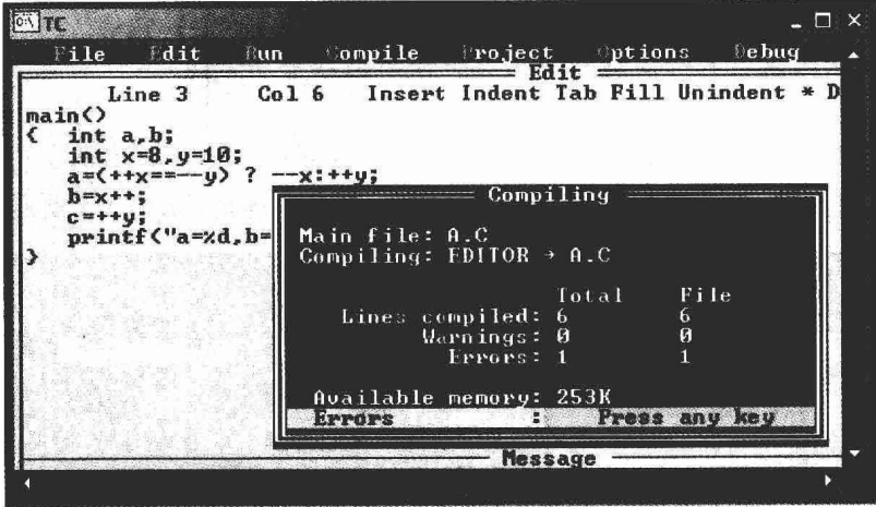
图 1-6 编译错误信息
