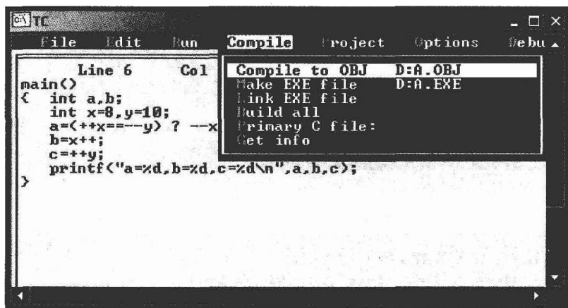
图 1-4 Compile 菜单中的编译选项
