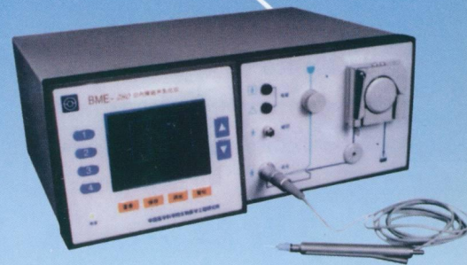
BME-280 白内障超声乳化仪
