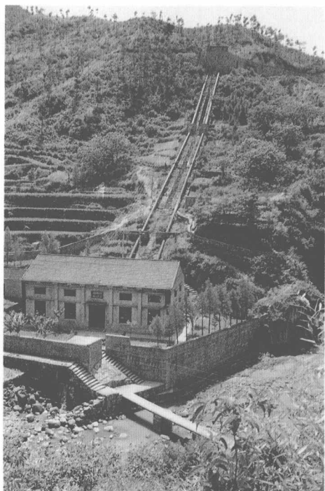
八〇电站
