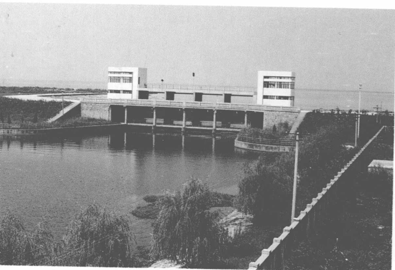
东进闸
