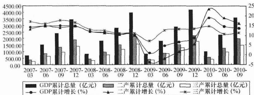
图 1 GDP 和二、三产业总量和累计增速走势图
