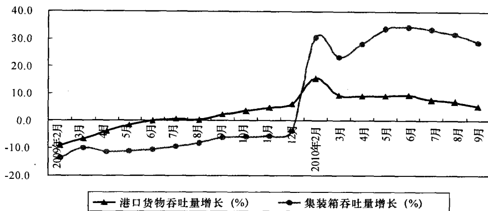
图2 集装箱及货物吞吐量累计增速走势图
