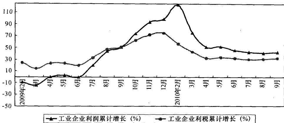
图4 规模以上工业企业利润和利税累计增速走势图
