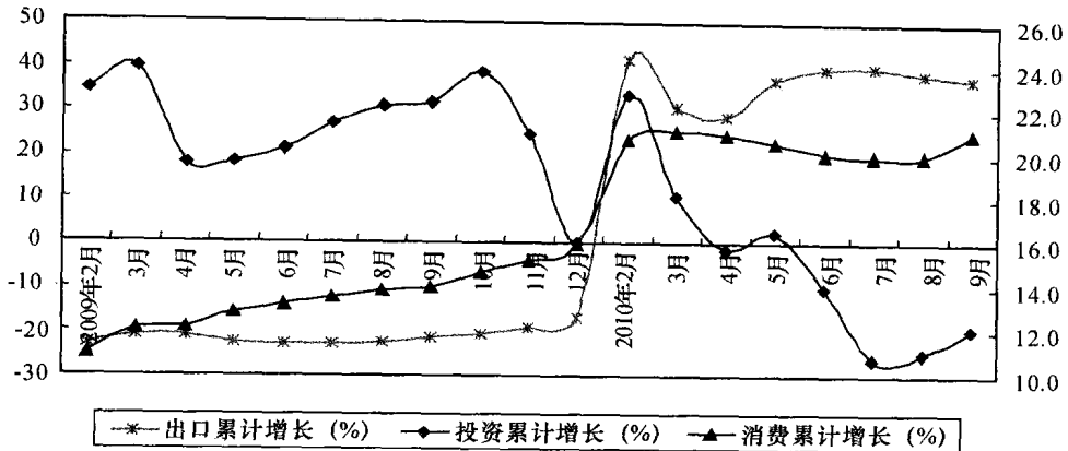
图3 投资、出口和消费累计增速走势图
