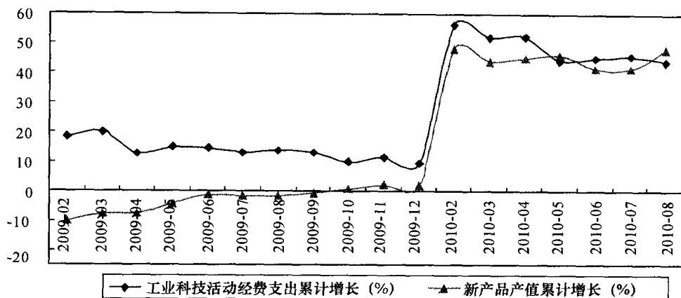
图6 宁波市工业科技活动经费支出及新产品产值增长趋势图
