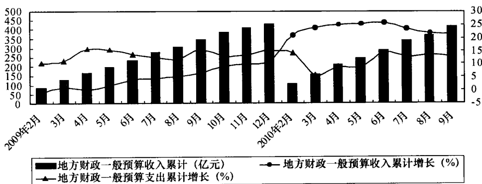
图 5 地方财政收入及支出累计增速走势图
