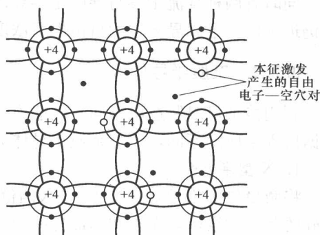
图 0.2.3 本征激发产生自由电子—空穴对
