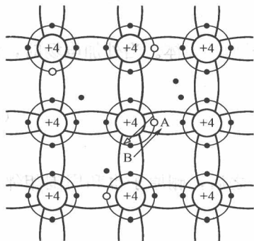
图 0.2.4 空穴运动
