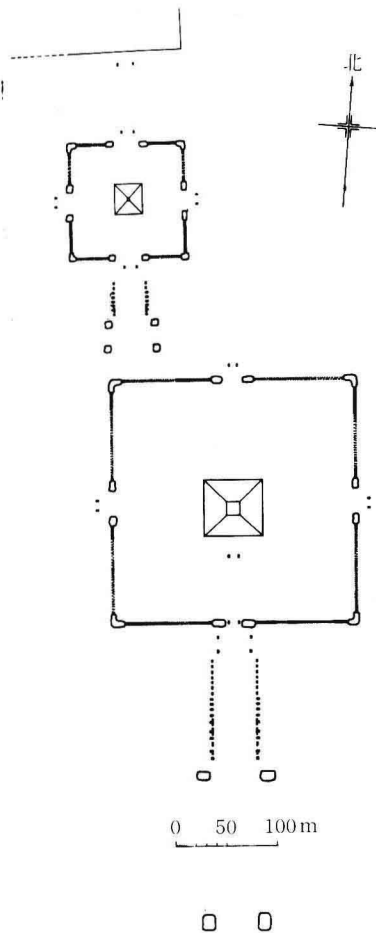
圖九 河南省鞏縣宋陵 永昭陵平面圖
