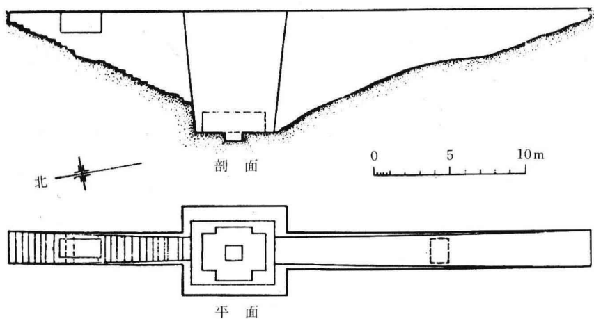
圖一 河南省安陽市後崗殷代墓平、剖面圖
