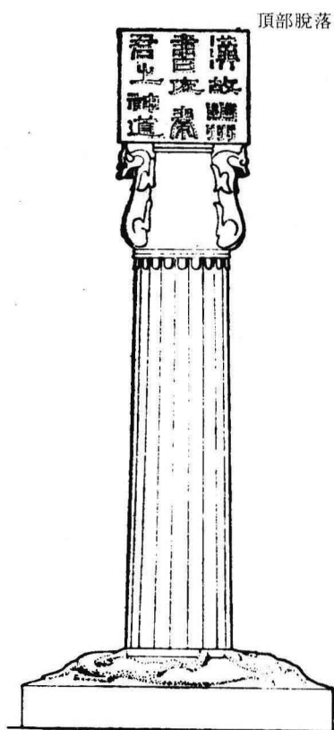
圖五 北京市西郊東漢秦君墓 墓表立面圖
