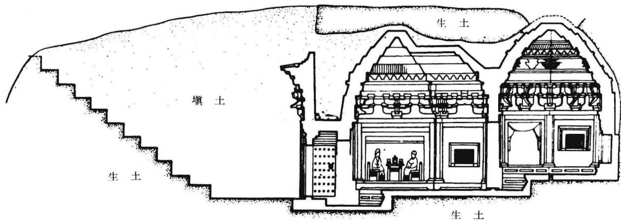
圖一一 河南省禹縣白沙宋墓第一號墓
