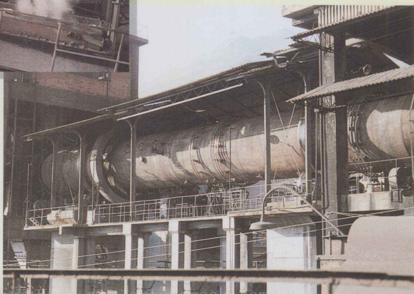
获国家级奖的云锡 100 吨/日难洗锡中矿回转窑高温氯化中间试验科研成果
