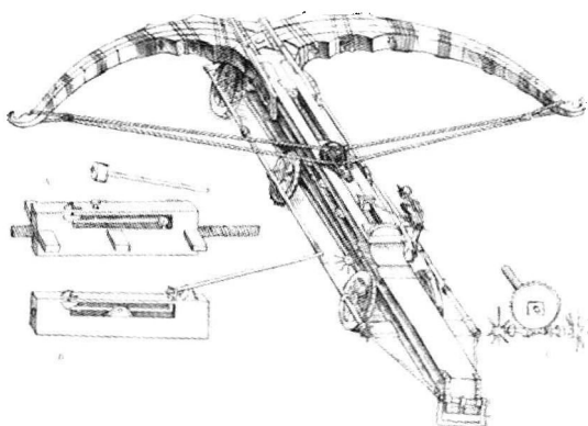
古代弩炮的构造
