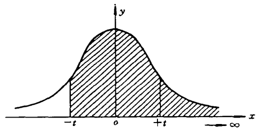
图 0-2 标准正态分布曲线
