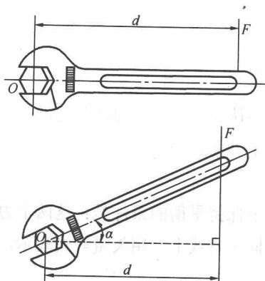
图 1-3 力矩
