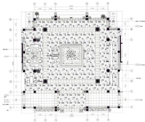
二层大堂平面详图
