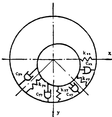
图 3 膜油力作用示意图
