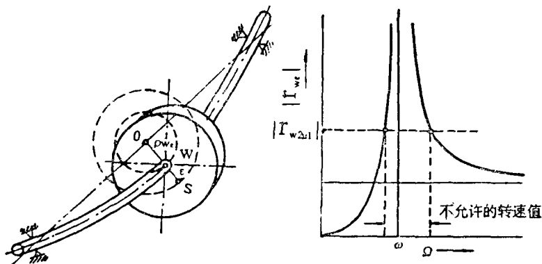
图 2 Jeffcott 转子
