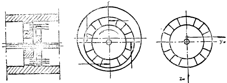
图 6 间隙蒸汽激励机理
