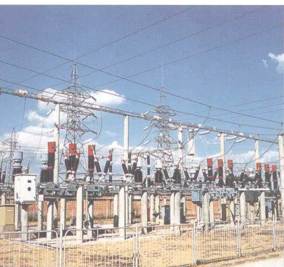
扎旗变电所
