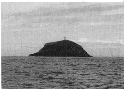
火山岛（福建南碇岛）
