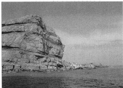
大陆岛（山东庙岛群岛）
