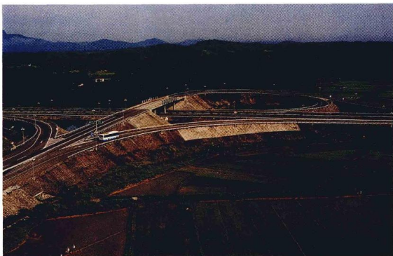
环岛东线高速公路
