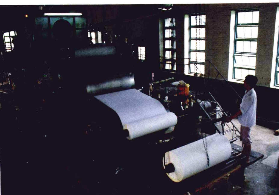
◁ 寻乌桂竹帽造纸厂造纸车间
