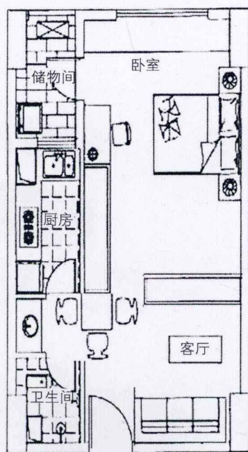
平面布置图
