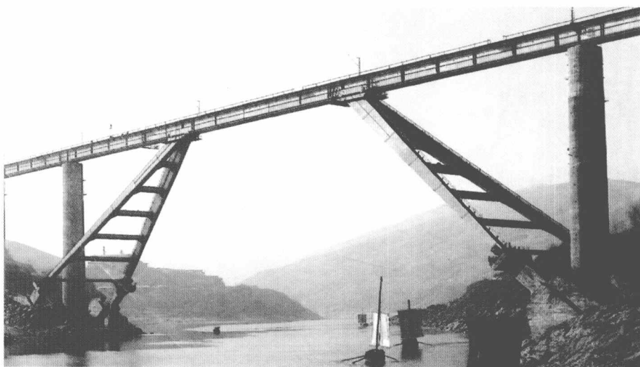
安康专用线斜腿钢构薄壁箱型钢梁桥(1982 年)
