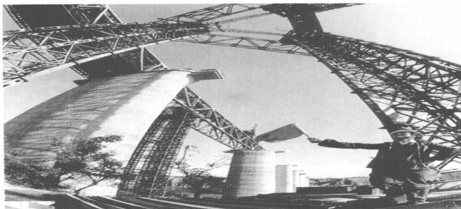
侯月铁路浚河大桥钢梁架设
