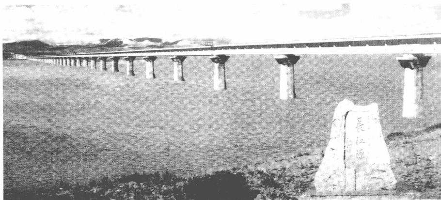
青藏铁路长江源沱沱河桥(2005 年)
