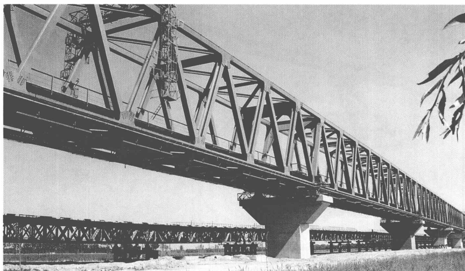
京九铁路孙口黄河大桥(1995 年)
