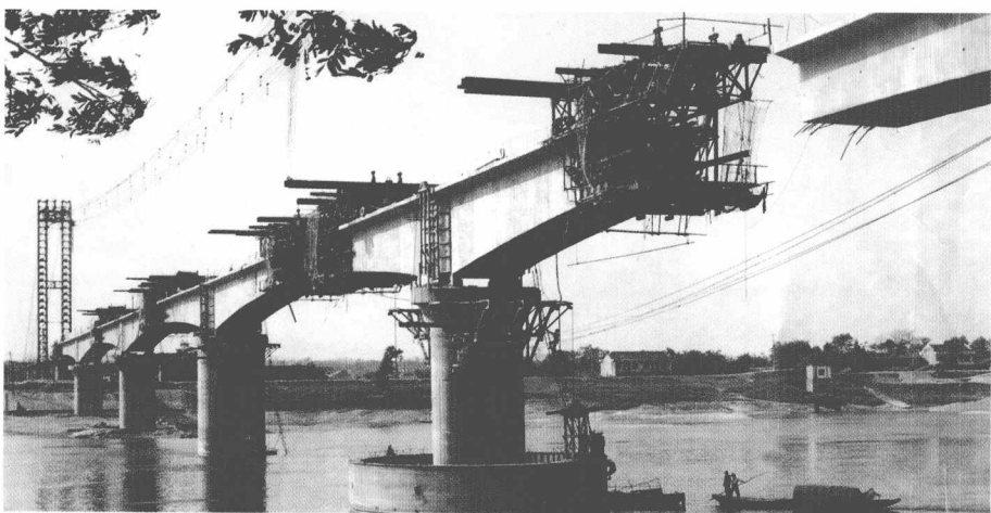
石长铁路资水桥连续梁施工
