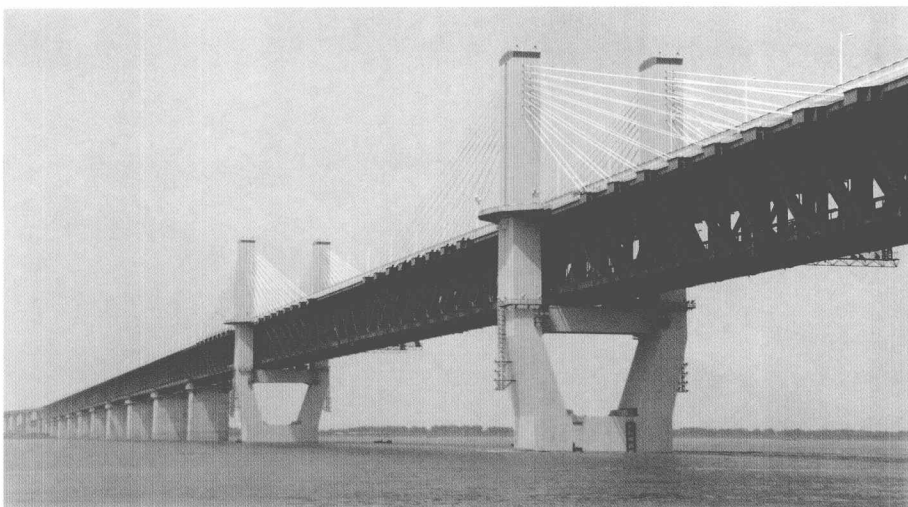
芜湖枢纽芜湖长江大桥(公铁两用,2000 年)
