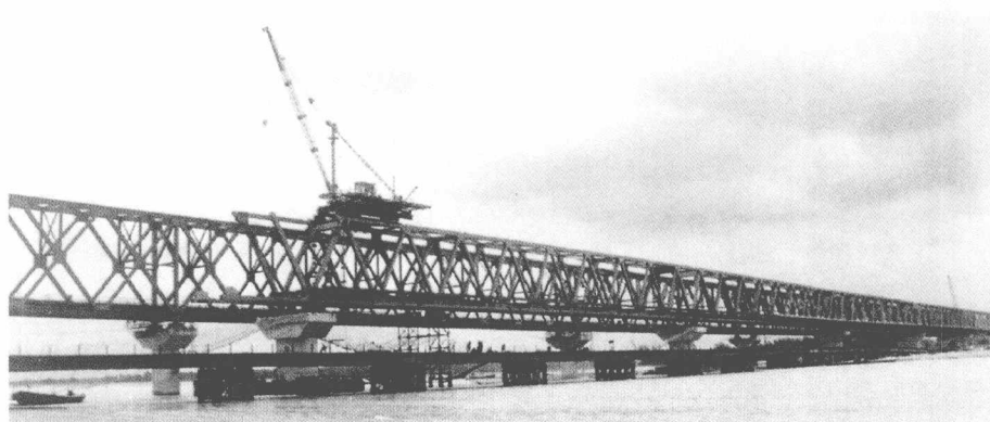
新菏铁路长东黄河二桥钢梁整体节点外拼装工艺
