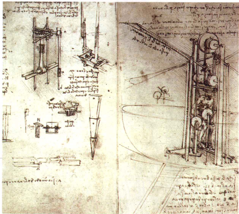
画家达·芬奇的挖壕机设计手稿
