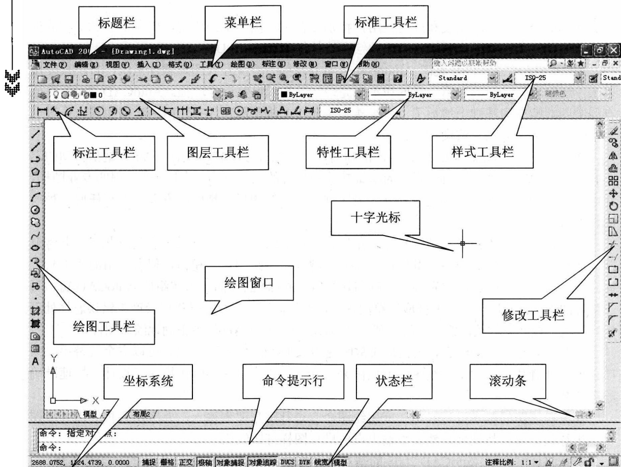
图 1-1 AutoCAD 2008 用户界面
