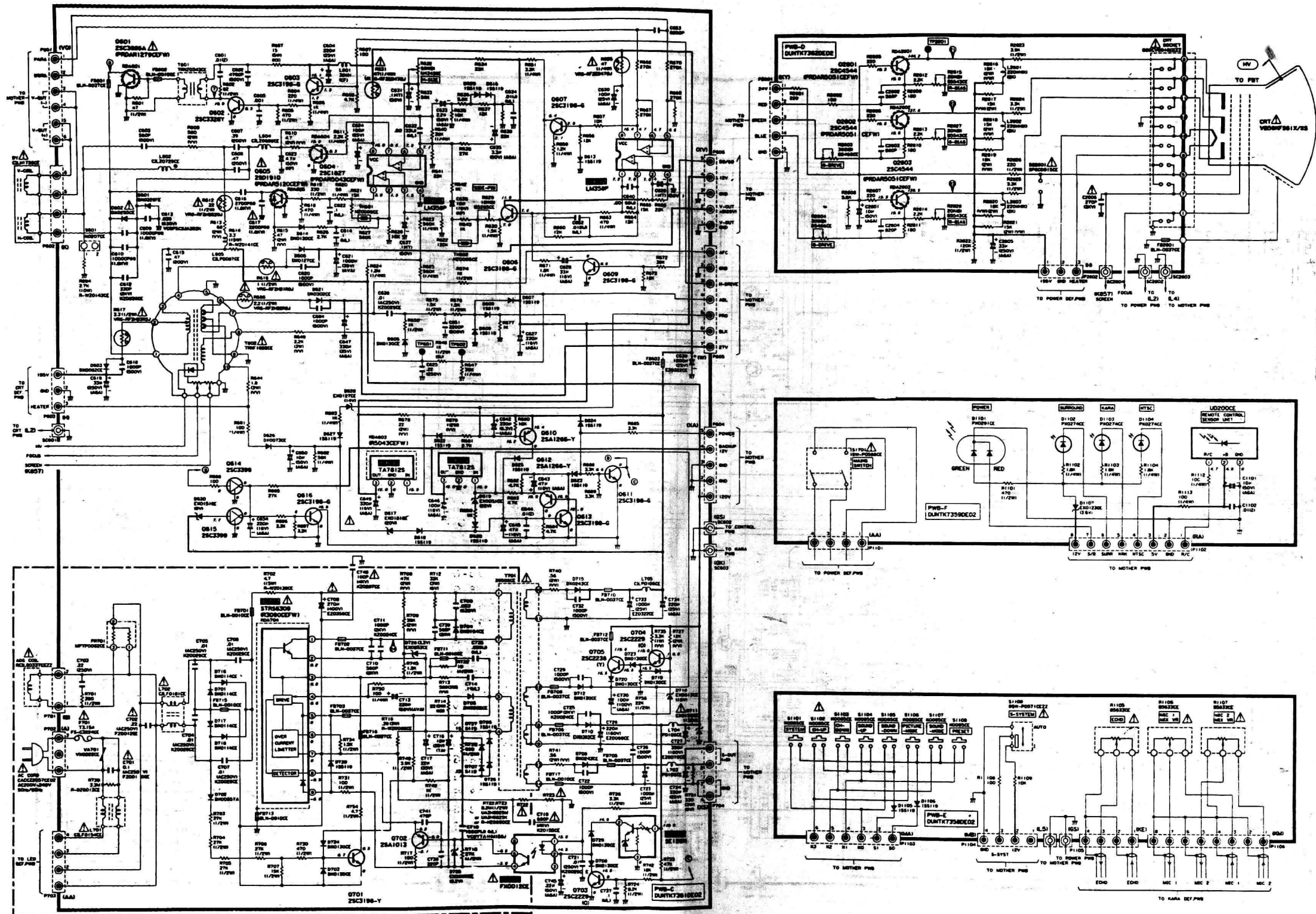
25A-K 型彩色电视机电路原理图(3)
