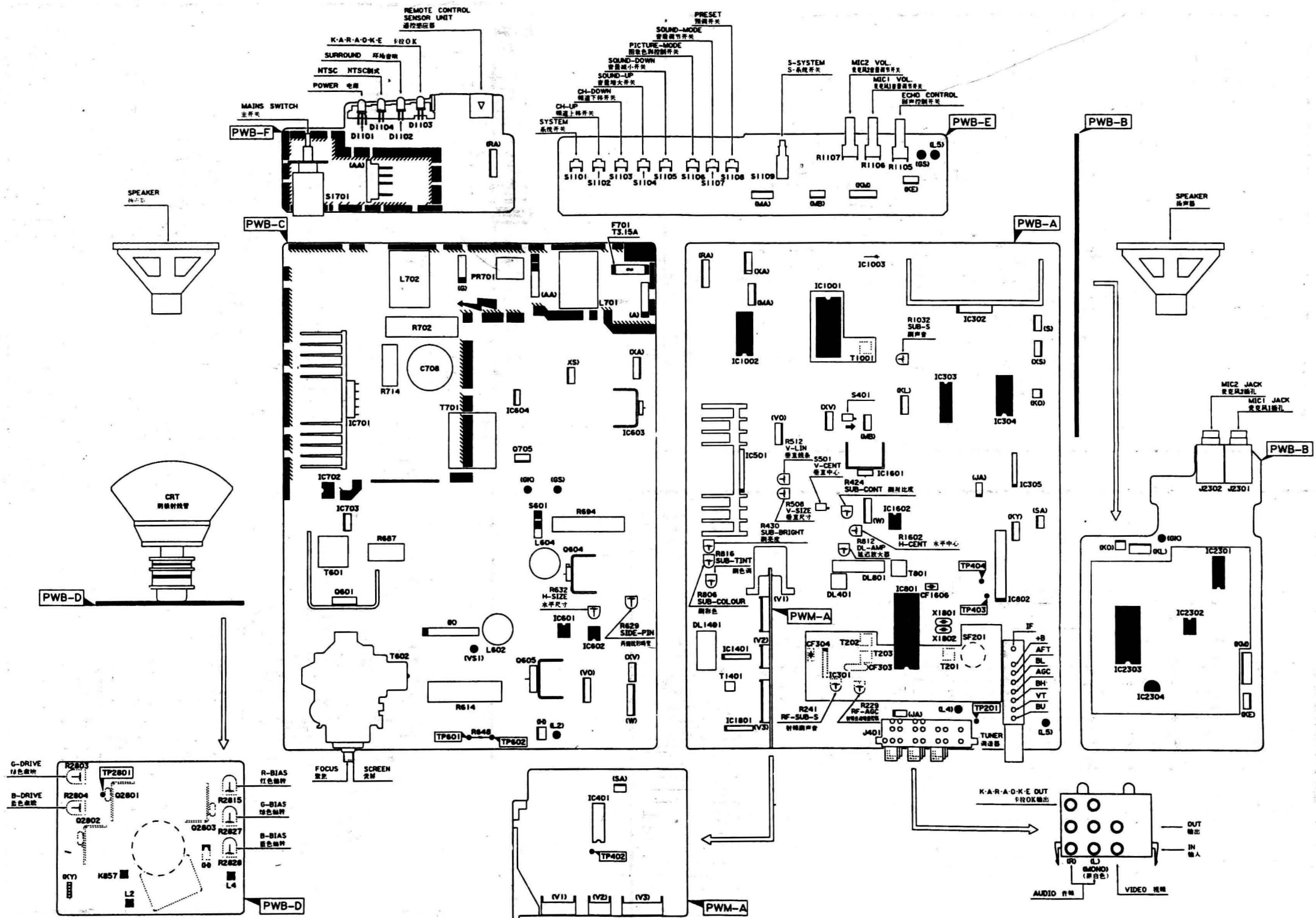
25A-K 型彩色电视机主要元件分部图
