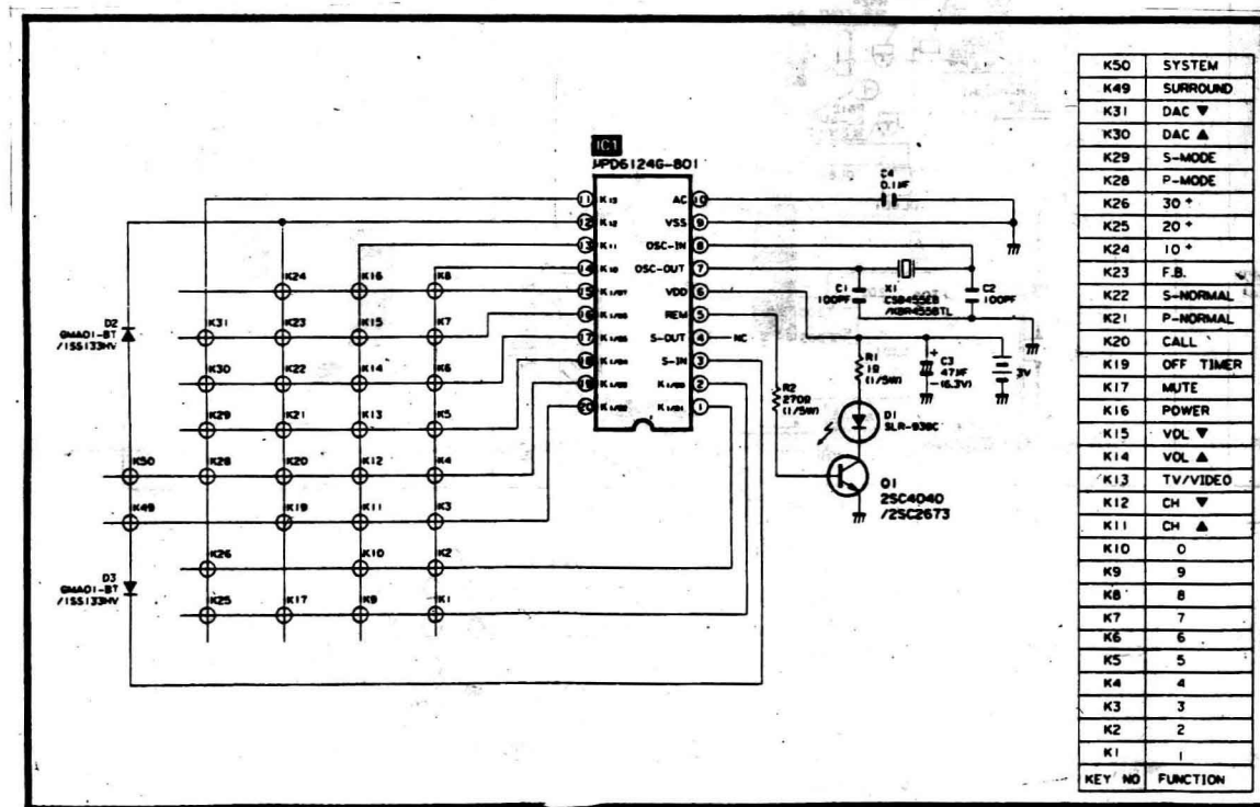
25A-K 型彩色电视机电路原理图(1)
