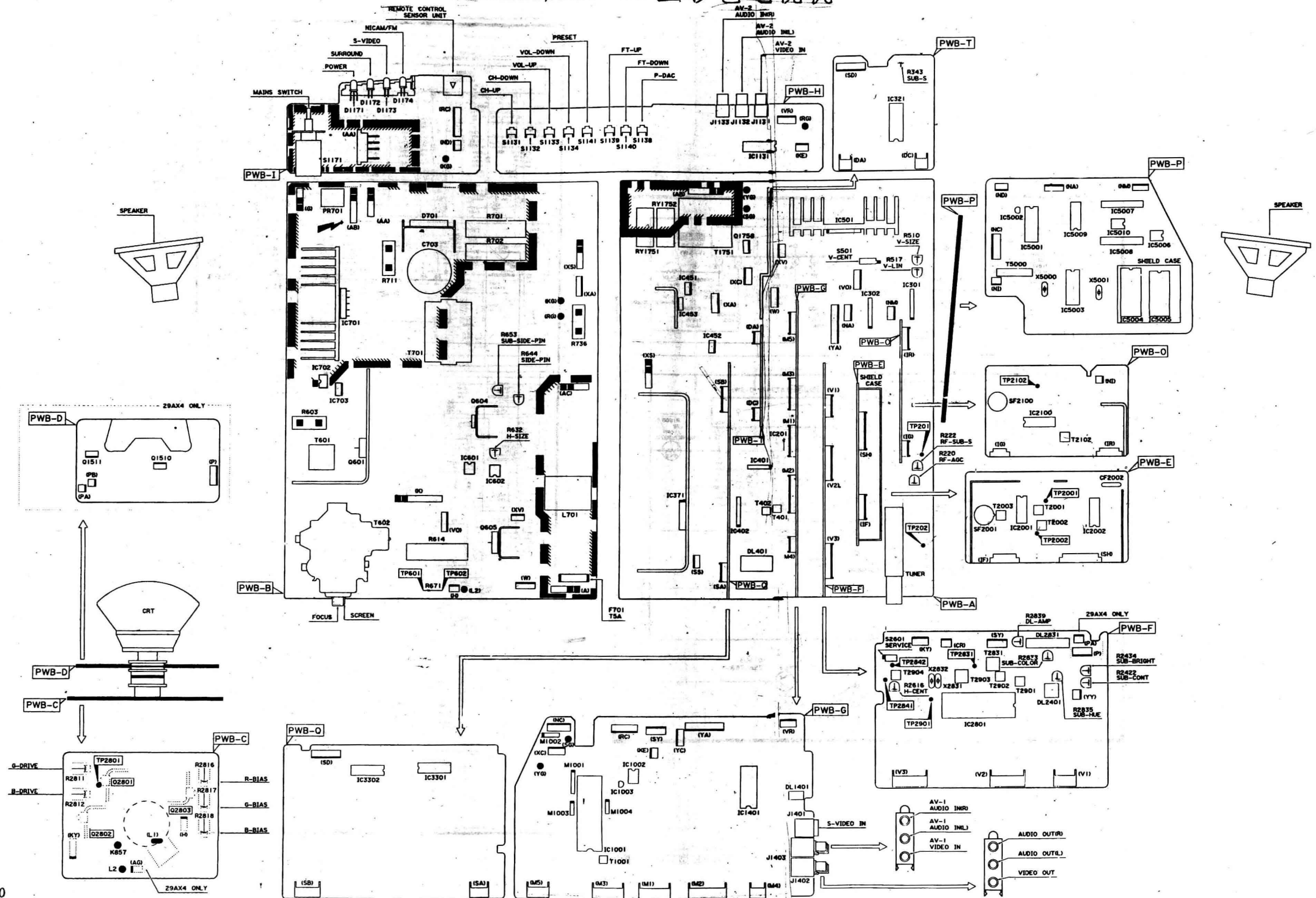
25Z×4/29A×4 型彩色电视机主要元件分布图
