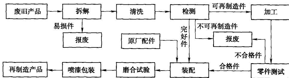
图 1-1 通常情况下再制造工艺流程
