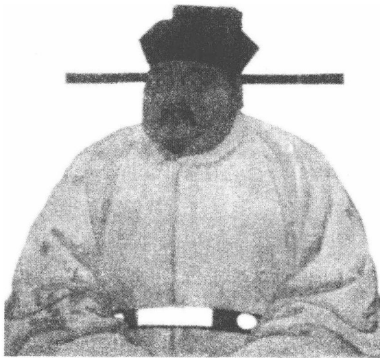
赵匡胤像
