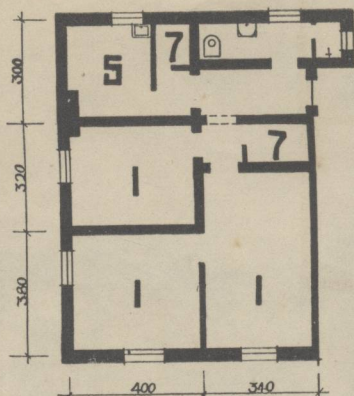
基本单元④
