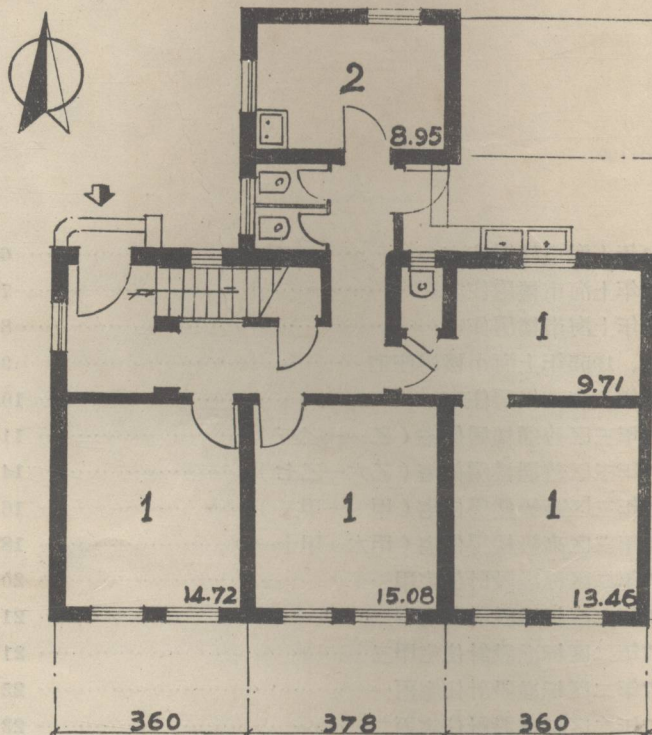
头层平面
