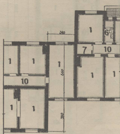
組合型連接基本補充平面
