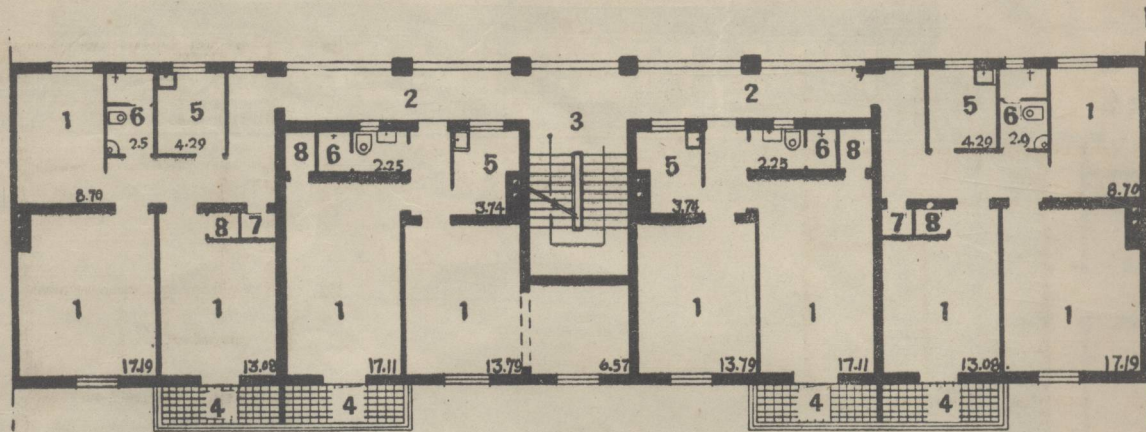
二、三层平面
