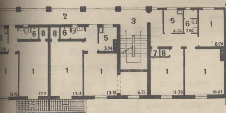
二、三层平面
