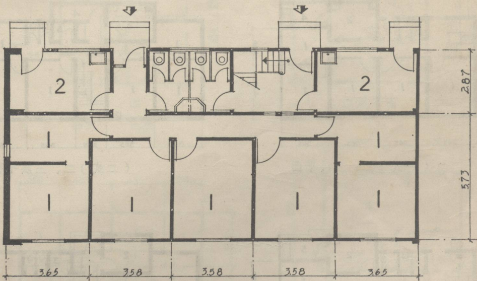
一层平面
