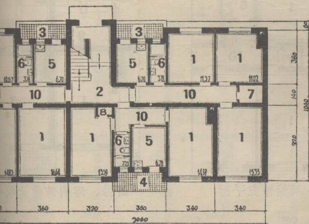
头层平面 2-3-3
