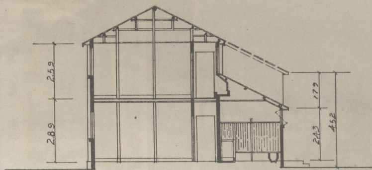
剖面
