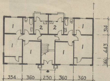
平面
