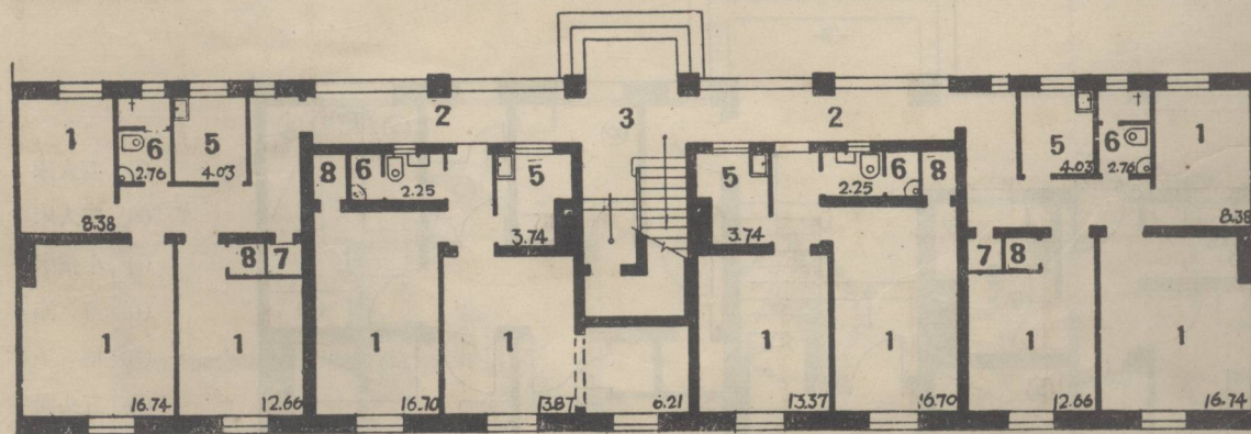
头层平面
