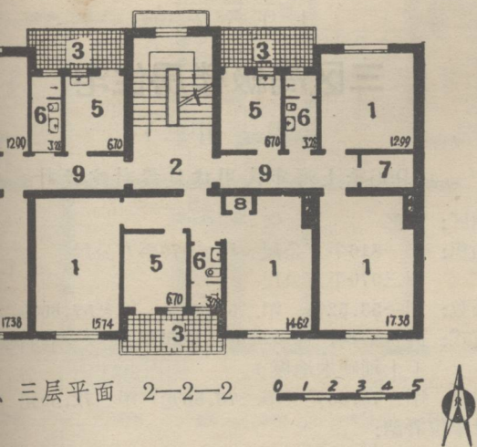
第三层楼梯間裝鉄爬梯通至閣頂
