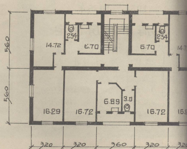
二、三层平面（五开间单元2-2-2）
