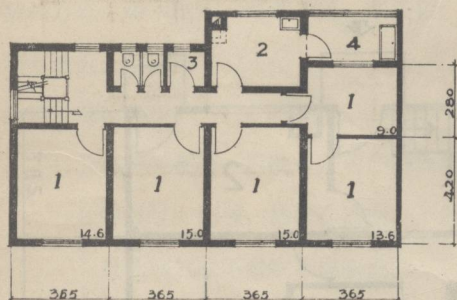
(一式) 二、三层平面
