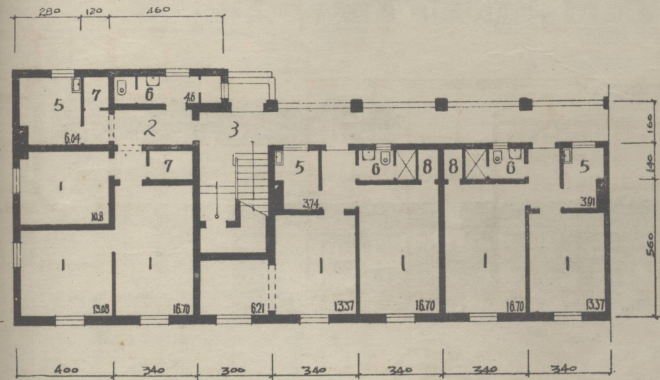
頭層平面 2-2-3
