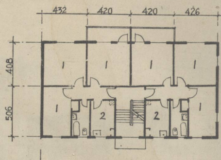
二层平面
