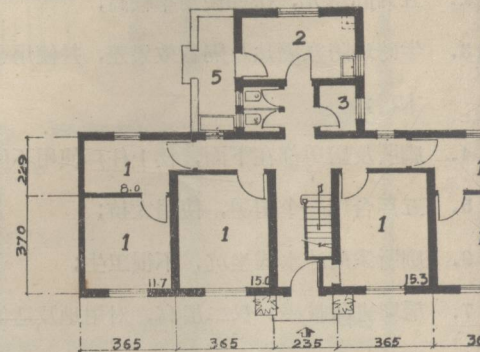
(三式) 头层平面
