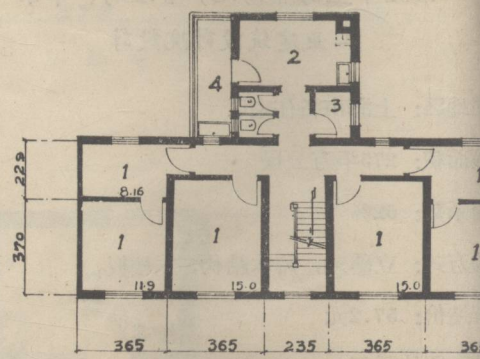
(三式) 二、三层平面
