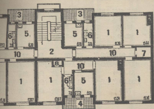
三层平面 2-3-3
