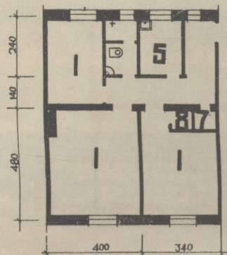
基本单元②
