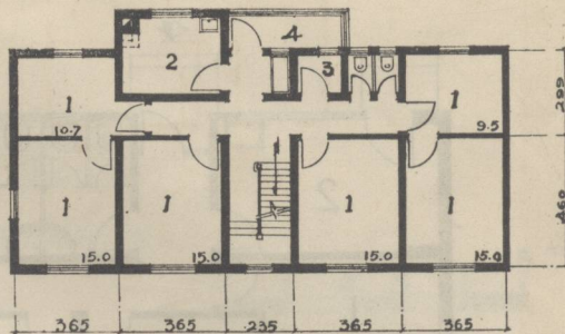
(二式) 二、三层平面
