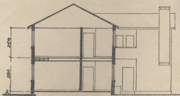
剖面
