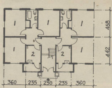
平面
