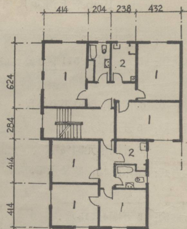
二层平面
