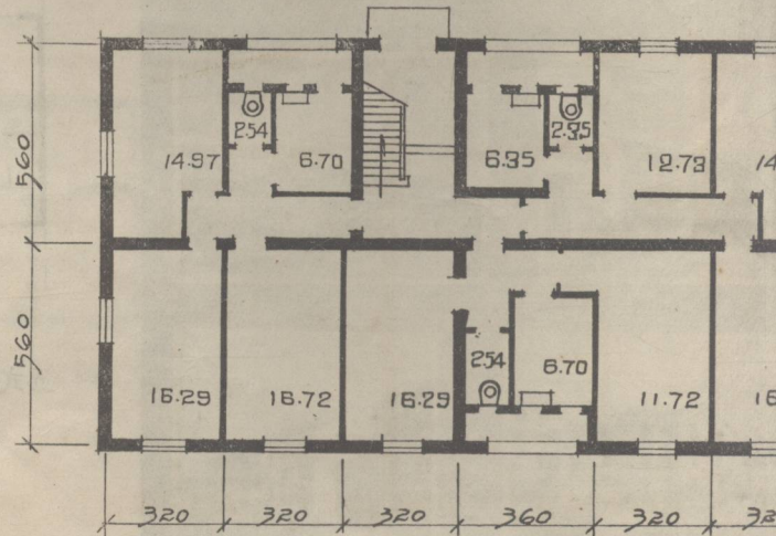
一层平面（六开间单元3-2-3）
