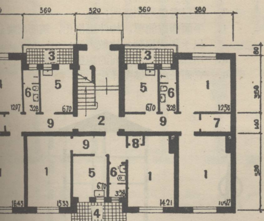
头层平面 2-2-2
