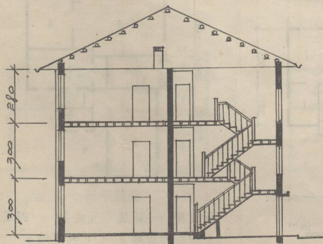
剖面
