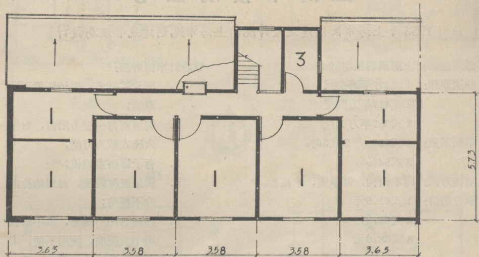
二层平面
