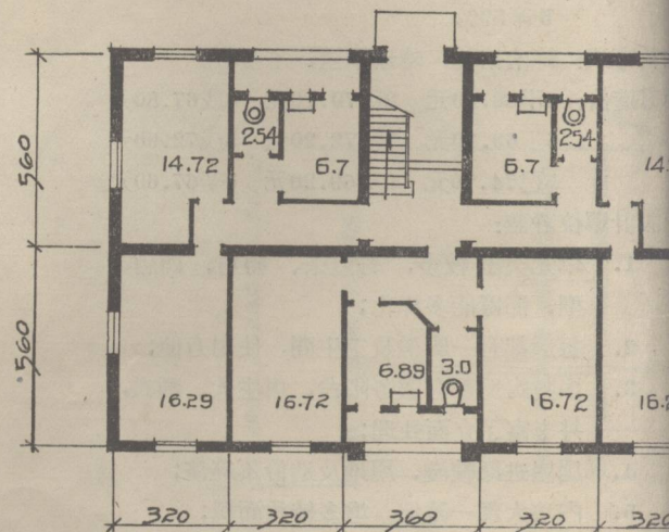
一层平面（五开间单元2-2-2）
