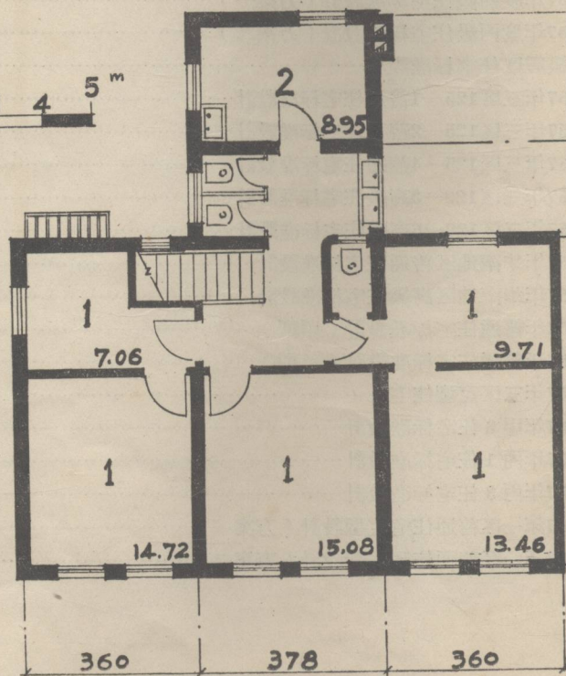
二层平面
