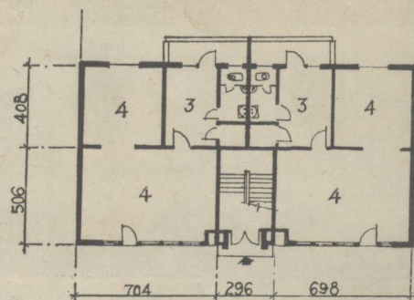
头层平面
