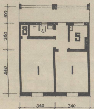
基本单元①
