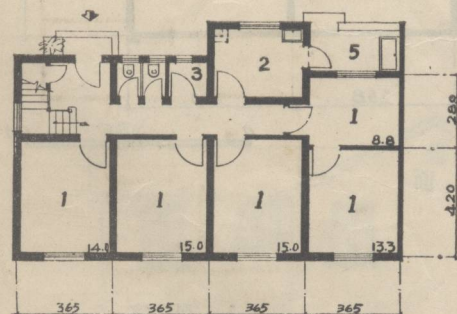
(一式) 头层平面
