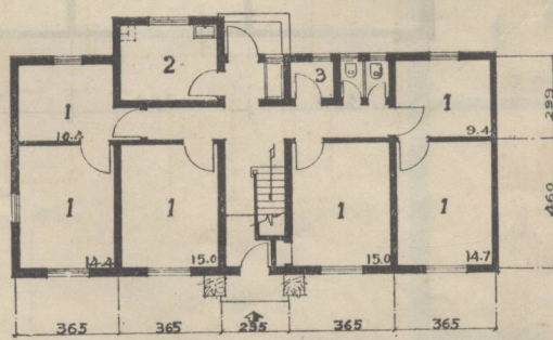
(二式) 头层平面
