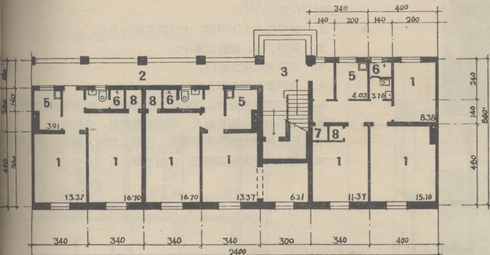
頭層平面 2-2-3
