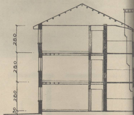
剖面
