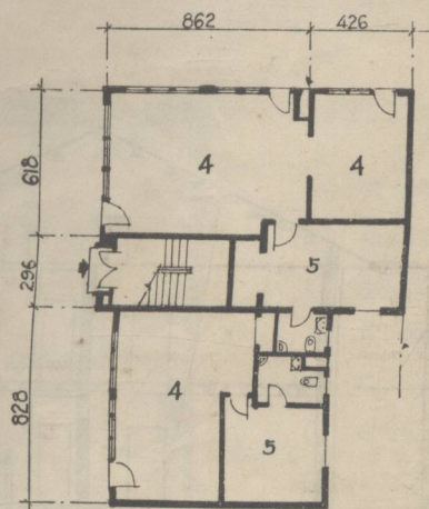
头层平面
