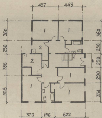
平面
