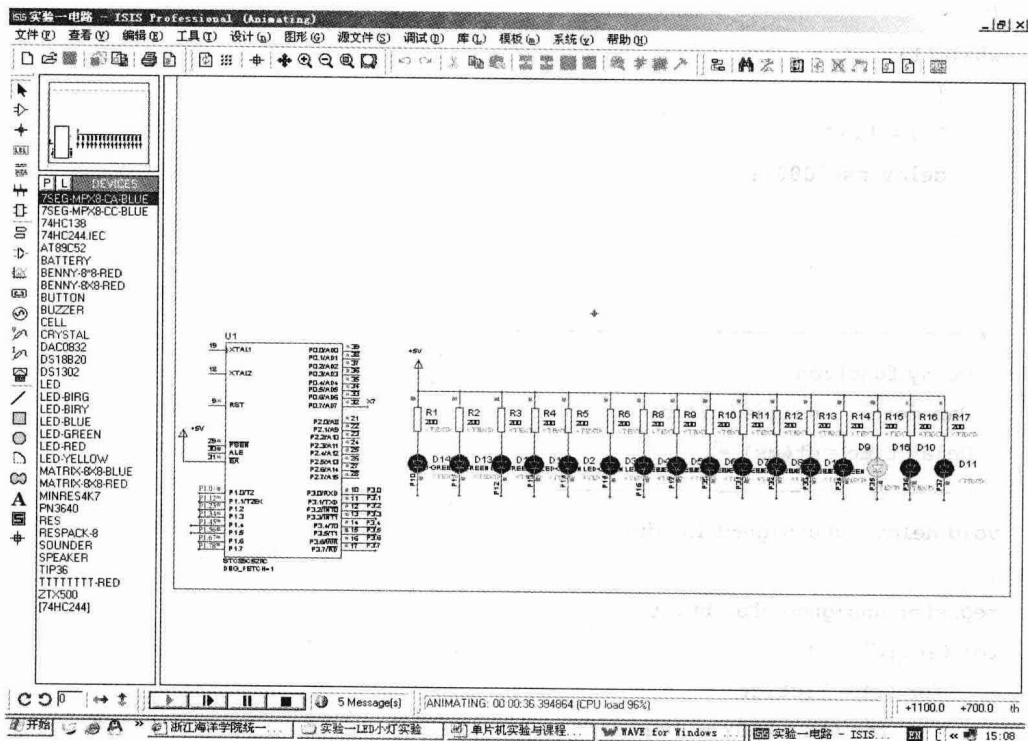
图 1.5 实验程序 1.4 的 Proteus 仿真效果
