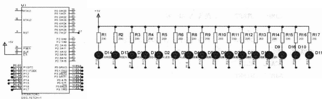
图 1.1 LED 小灯实验仿真硬件电路
