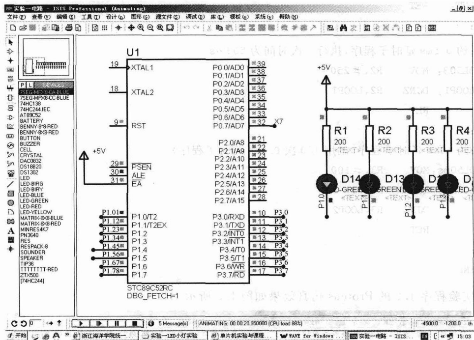
图 1.2 实验程序 1.1 的 Proteus 仿真效果
