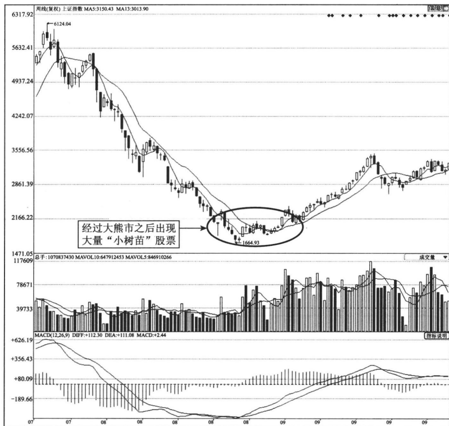
图 1-3 上证指数 2007—2010 年周 K 线走势图(一)
