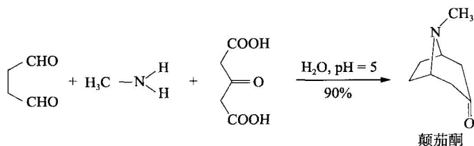
图 1-1 Robinson 报道的颠茄酮一步合成法
