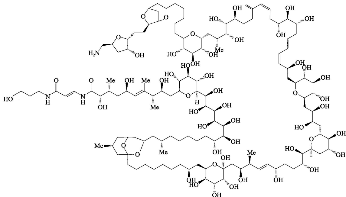
岩沙海葵毒素 (Palytoxin) 的结构
