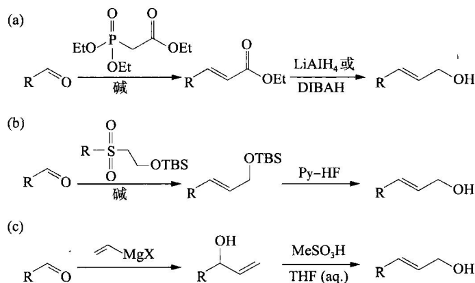
图 1-2 末端烯丙醇的三种常规合成方法(合成效率低)
