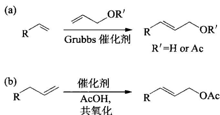
图 1-3 末端烯丙醇的高效合成方法(合成效率高)
