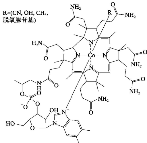
维生素B 12 的化学结构
