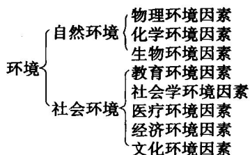
图 1-1 环境的分类
