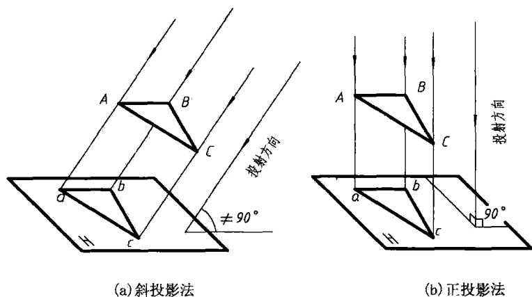
图 2 平行投影法
