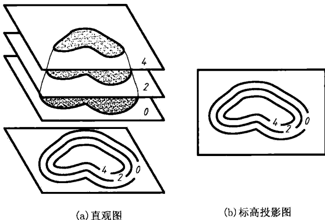
图 5 标高投影图
