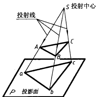
图 1 中心投影法
