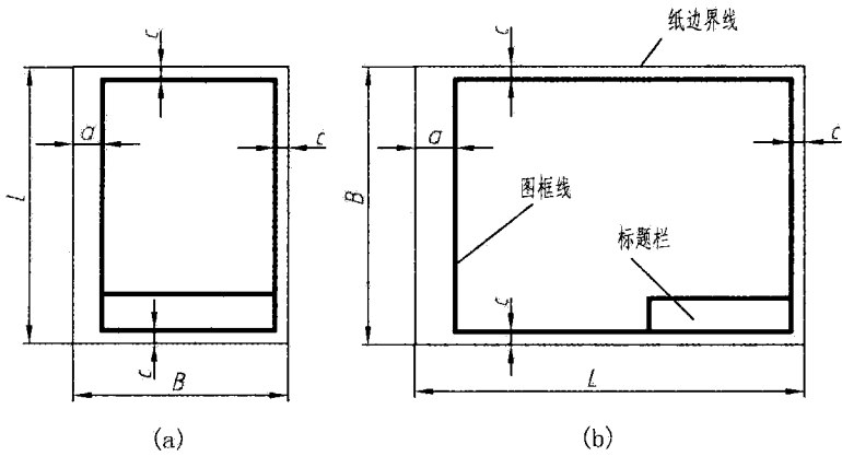
图 1.2 图框格式(二)
