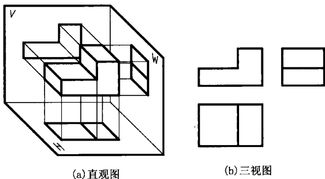
图 3 正投影图
