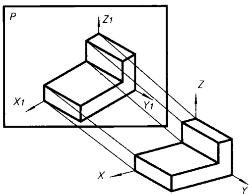
图 4 轴测投影图
