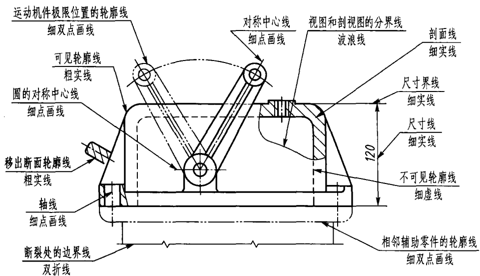
图 1-8 图线应用举例
