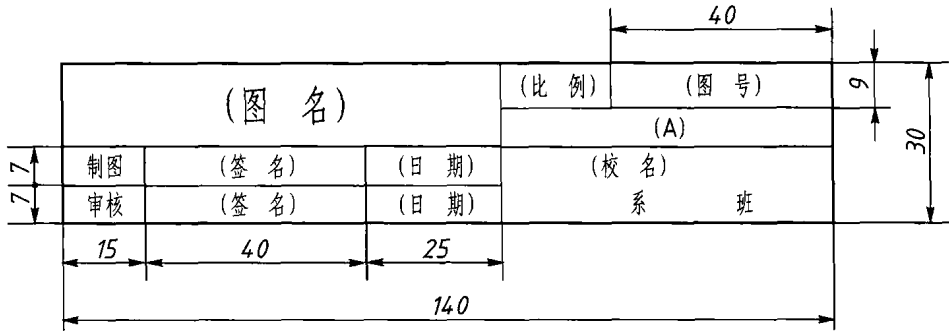
图 1-3 推荐使用的标题栏格式
