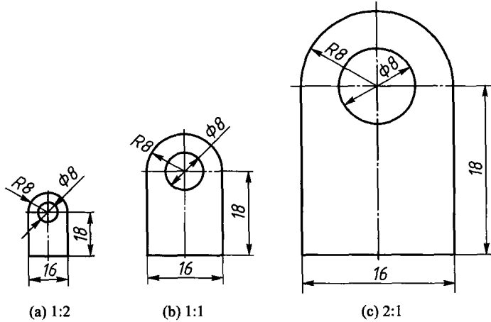
图 1-5 用不同比例画出的图形
