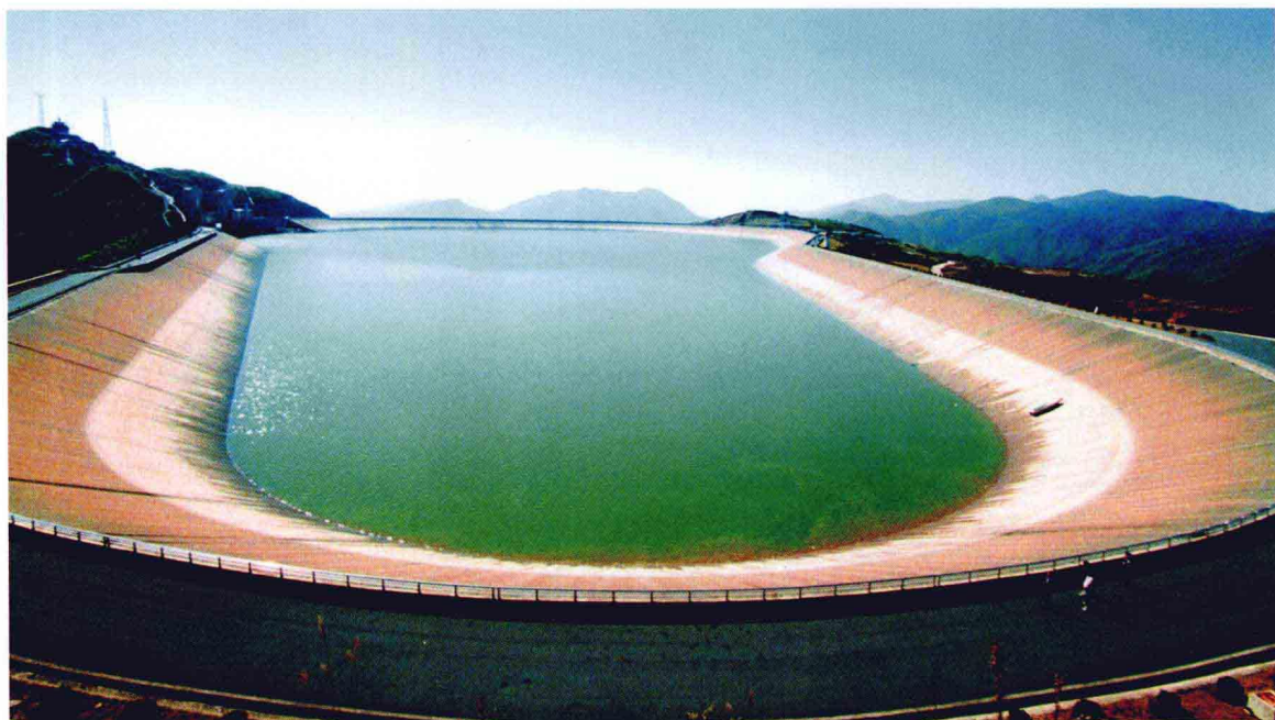
▲ 安吉天荒坪抽水蓄能电站于1996年开始动工兴建，2000年竣工投入使用，是亚洲最大的抽水蓄能电站。该电站雄伟壮观，堪称世纪之作。
