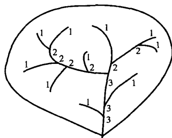
图 1-1 流域和水系 1~3—河流的级别
