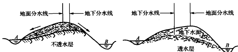
图 1-2 流域地面和地下分水线示意图
