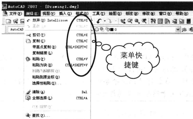
图 1-6 菜单快捷键
