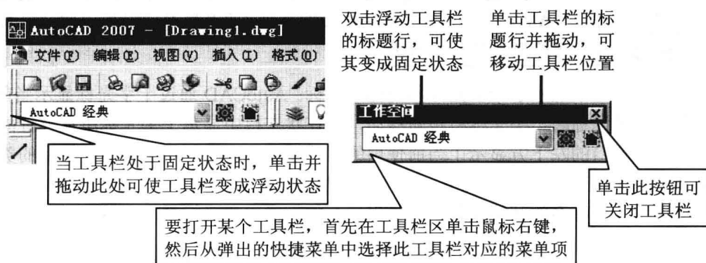
图 1-4 工具栏操作
