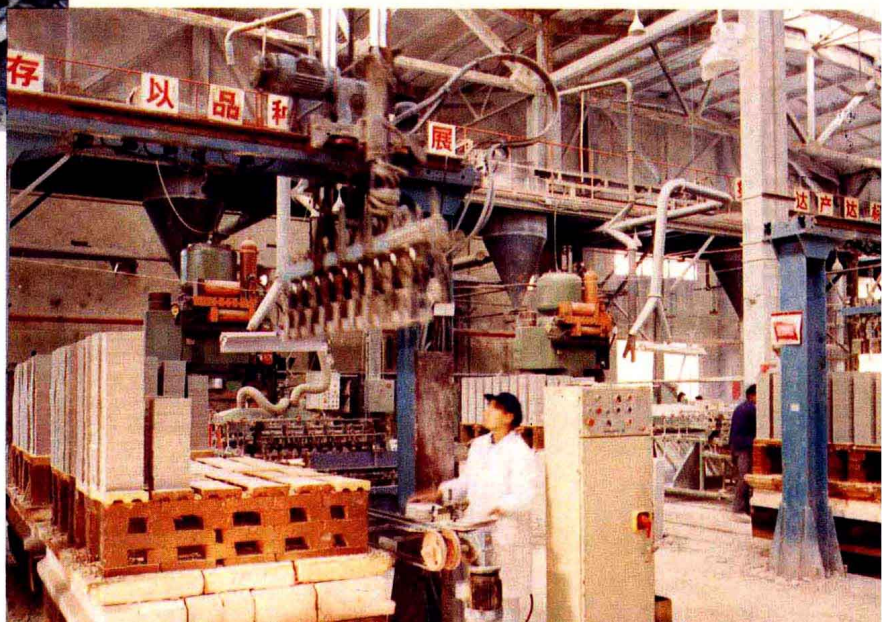
釉面砖生产作业线 ▶
