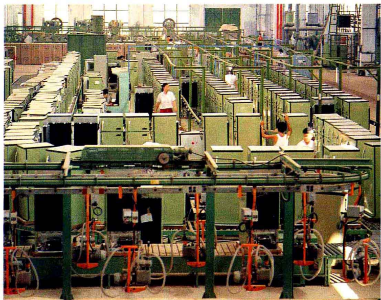
▼ 华意电冰箱生产作业线 (金向东摄)
