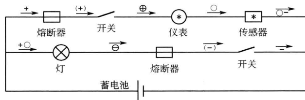
线路符号表达示意简图
