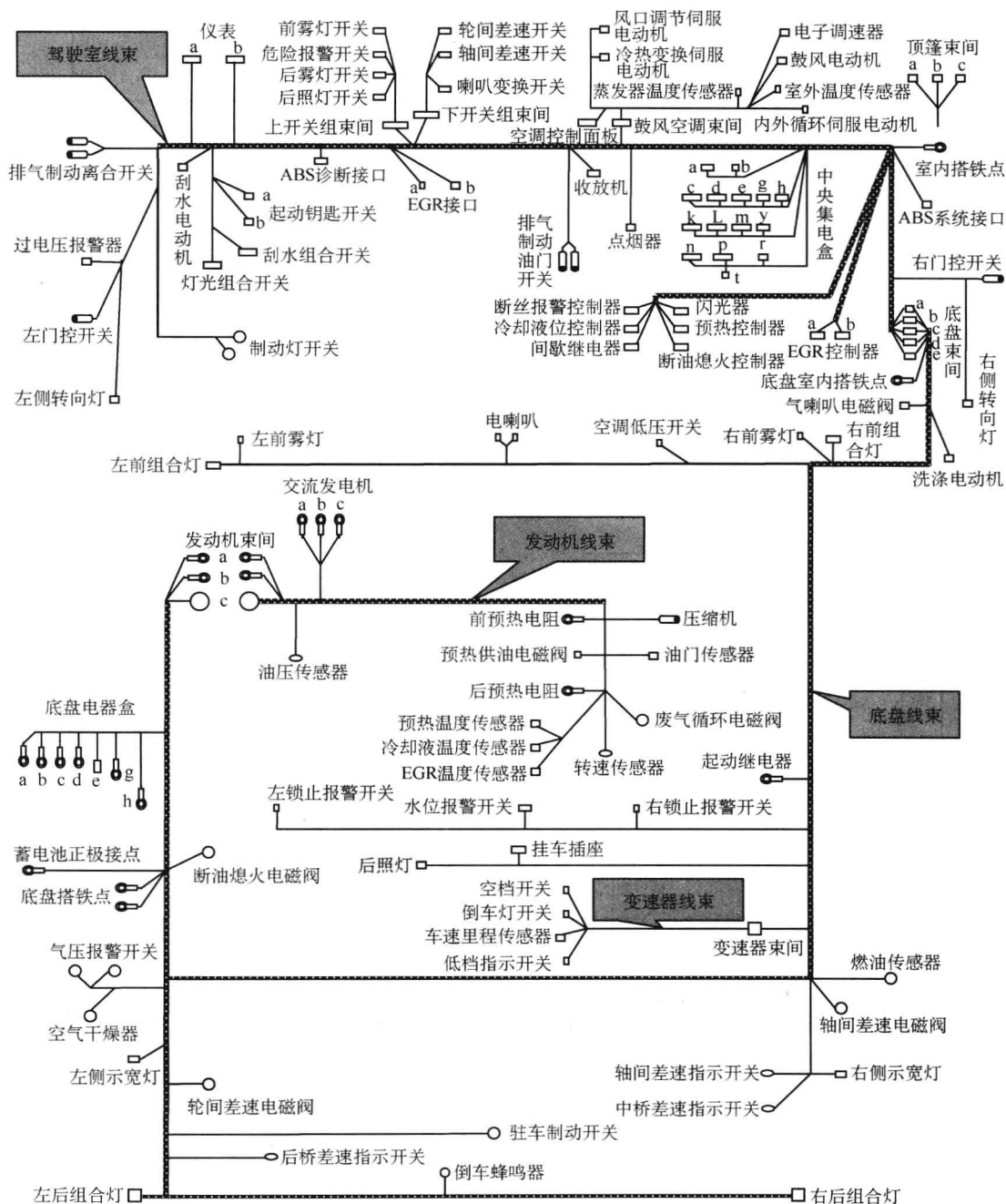
图 1-1 解放新大威 CA4228P2K2 型平头柴油牵引车线束布局图
