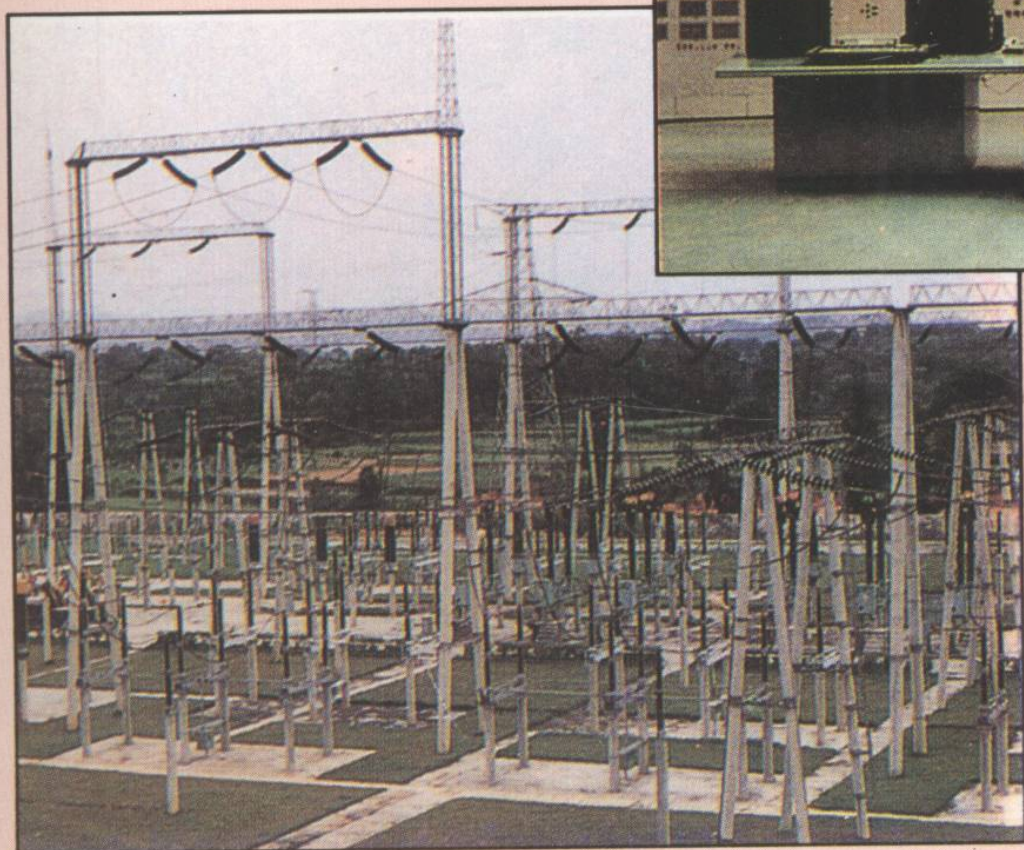
设在荔城镇的220千伏输变电站
